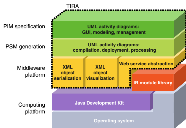
Abbildung 7: Die Schichtenarchitektur von TIRA setzt auf einer Rechnerplattform auf. Die IR-Modul-Bibliothek ist nicht Teil von TIRA, sondern steht für eine offene und erweiterbare Menge von IR-bezogenen Algorithmen und Datenstrukturen.
